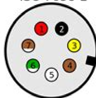
ISO 7638-2
