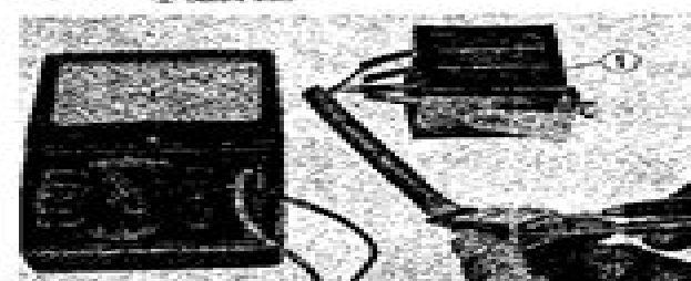
Fig. 153 Selenium rectifier continuity test ① Selenium rectifier
