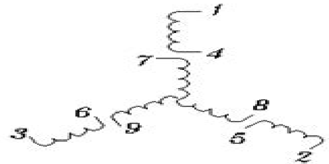
Y or STAR
