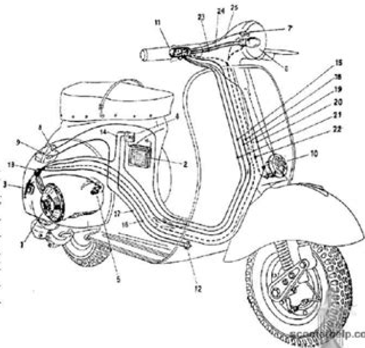
Fig. 11.—Instalación eléctrica sobre la moto.
