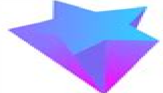
star pyramid
