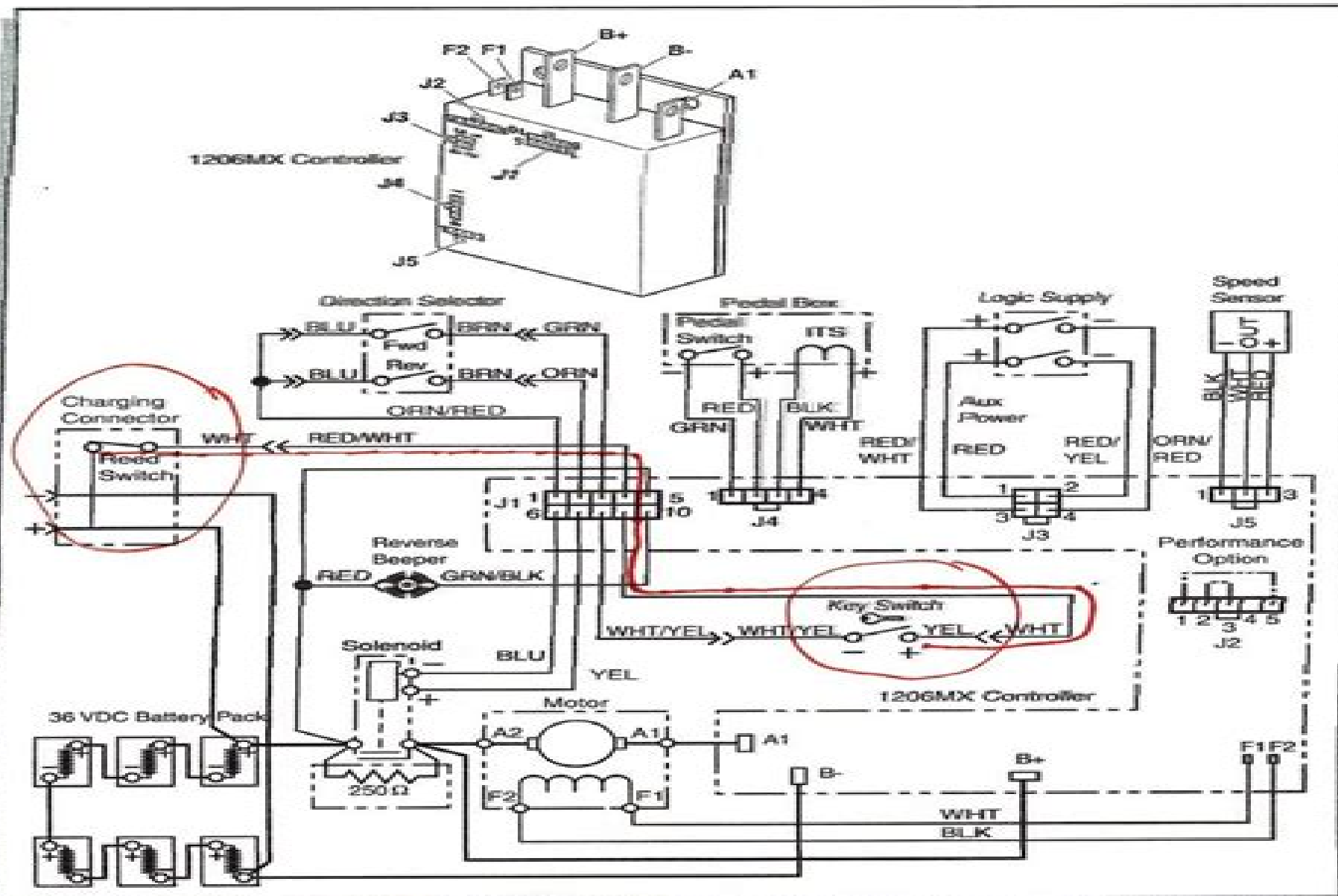
Fig. 9 Wiring Diagram
