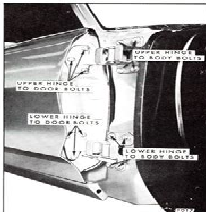
Fig. 1D33—Front Door Hinge Attachment
