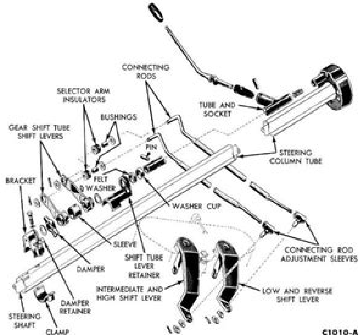
FIG. 1—Typical Gear Shift Linkage
