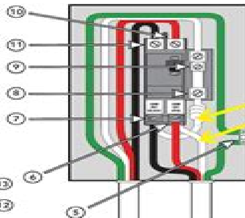
G.F.C.I Breaker Box
