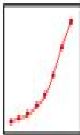
AIEE moleculars
