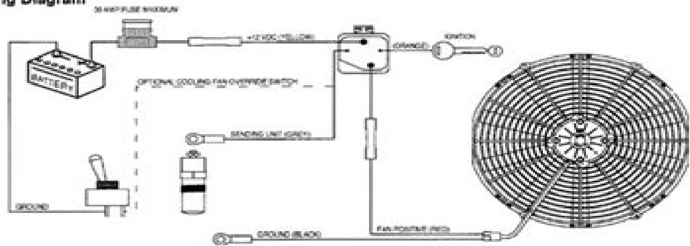
Multiple Fan Wiring Diagram
