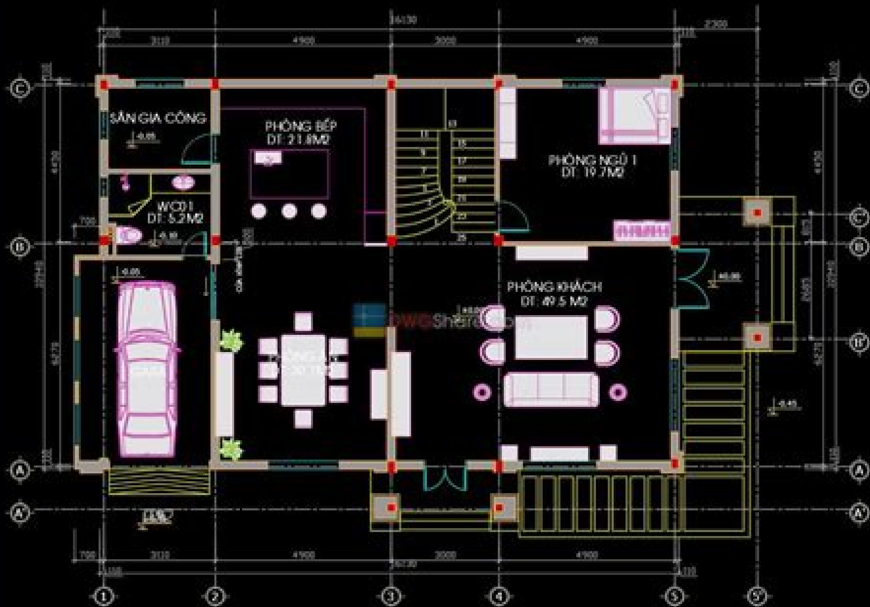
MẶT BẰNG HIỆN TRẠNG TẦNG 1
